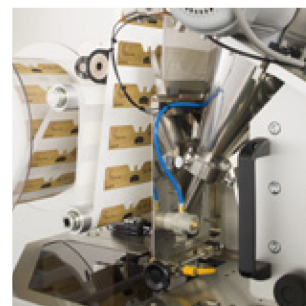
オーガー充填装置(オプション)
