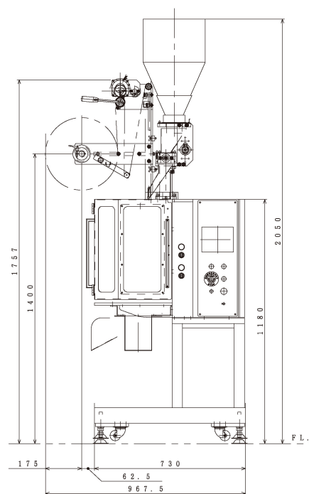
FP-CS標準仕様(マス計量)
