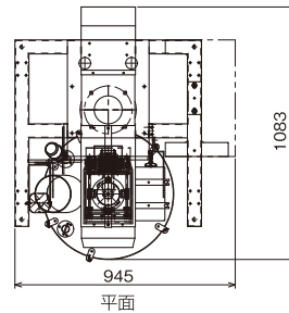
外観図(FAF-60LS)
