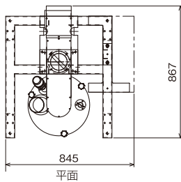
外観図(FAF-14LS)
